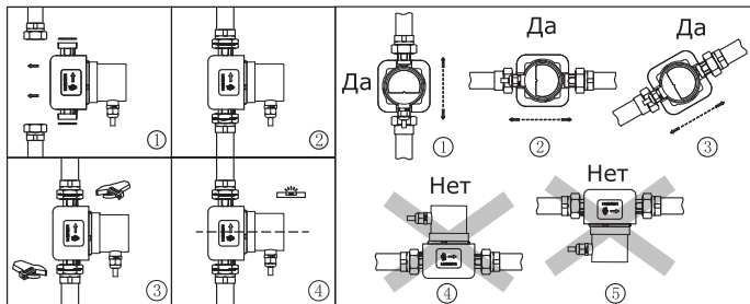
Рис.3 Установка циркуляционного насоса
