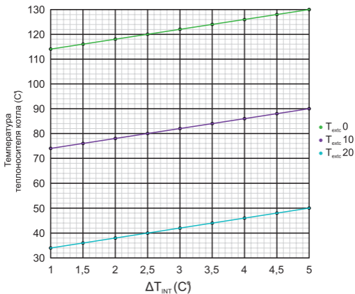
Рис. 11 Тепловая кривая с K_{somr}=8
