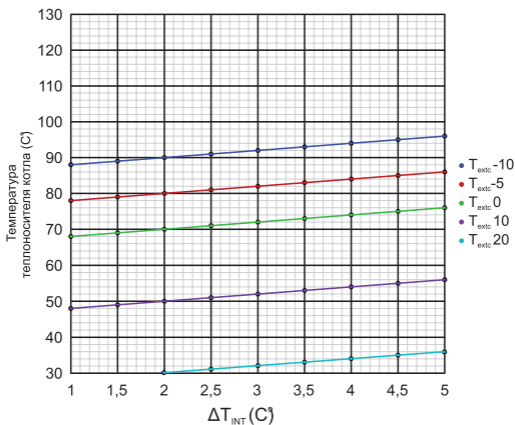
Рис. 12 Тепловая кривая с K_{somr}=4
