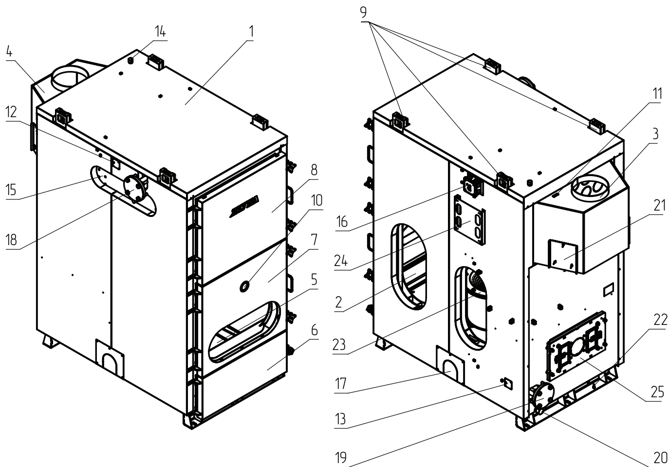
Рис.2 Конструкция теплообменника котла ZOTA Robot
