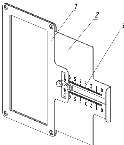
Рис.23 Заслонка вентилятора
