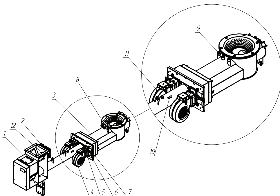
Рис.5 Механизм подачи топлива с горелкой котла
