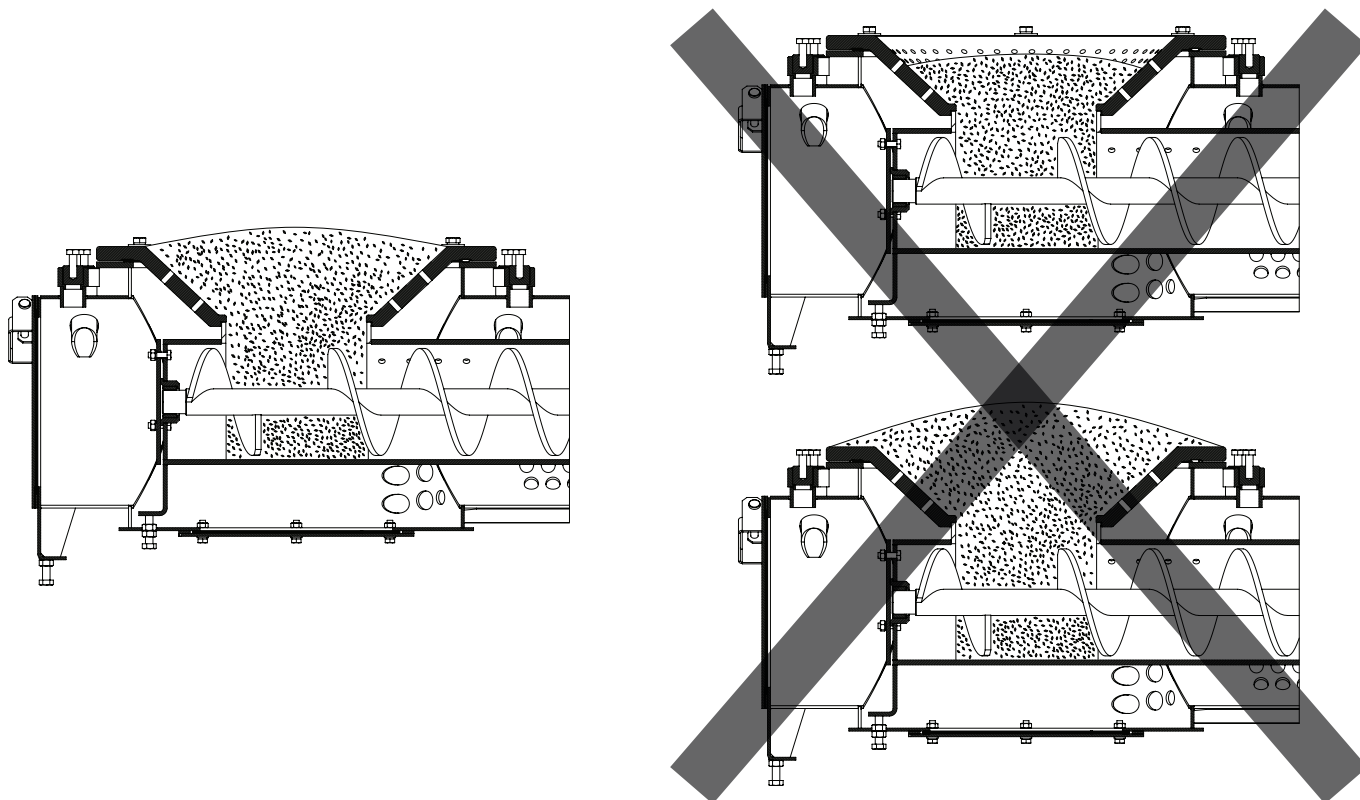
Рис.22 Настройка уровня топлива при горении
