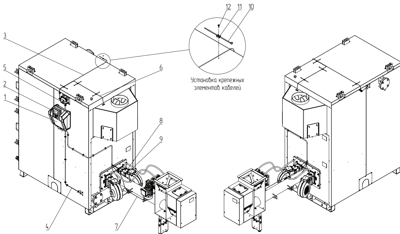
Рис.21 Схема подключения контроллера и укладки кабелей для котлов стационарного исполнения
