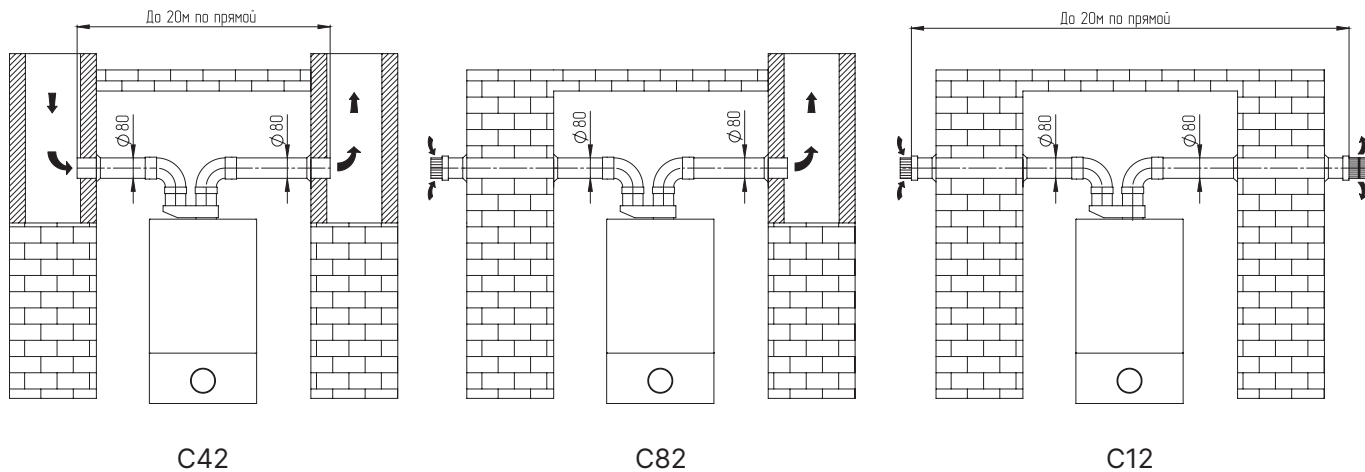
Рис. 23 Варианты монтажа раздельной системы дымохода горизонтально
