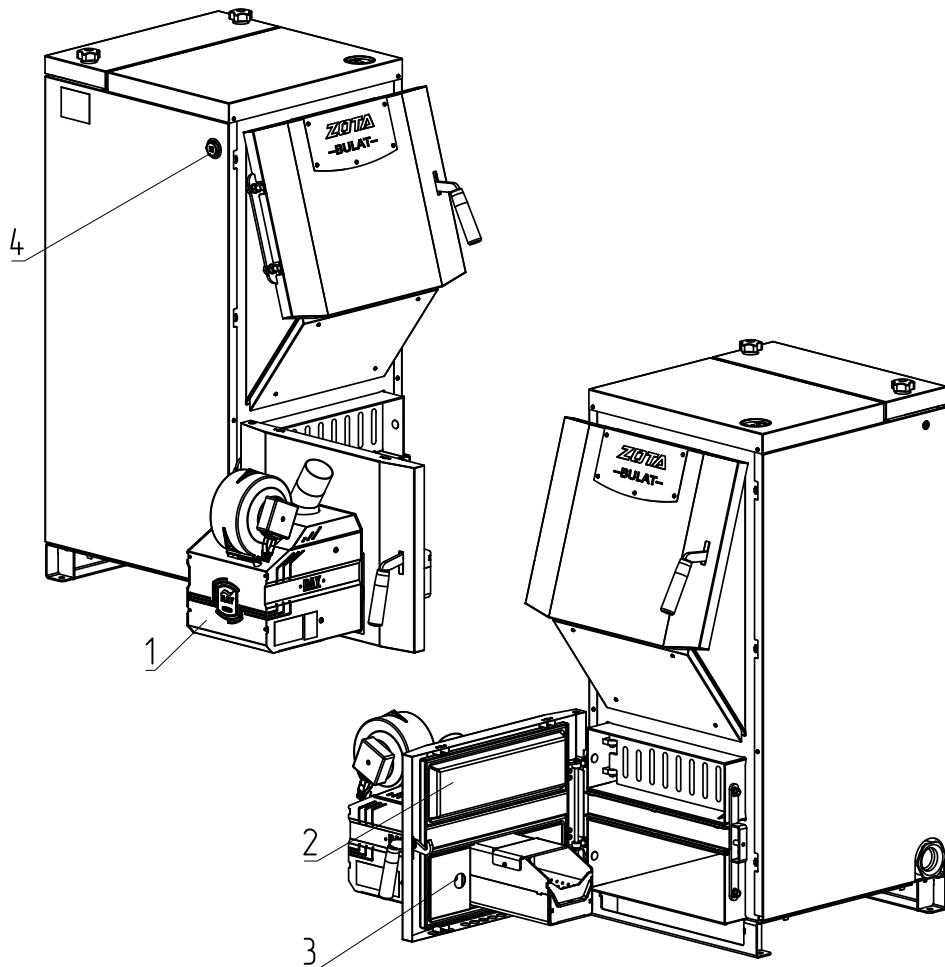
Рис.9. Порядок установки пеллетной горелки на твердотопливные котлы ZOTA Bulat 18, 23, 28.
