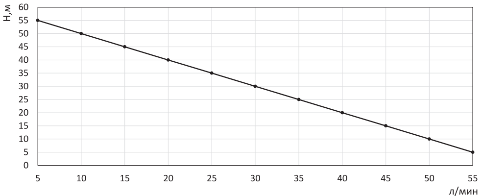
Рис. 1 Расходно-напорная характеристика насосной станции
